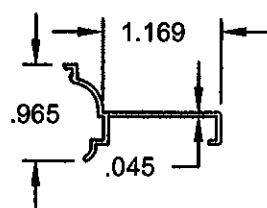
(106) #8026A 6063-T5 SL BACKBEAD
