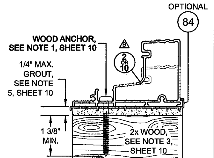
OPTIONAL DOOR SILL (SUBSILL TO WOOD)
