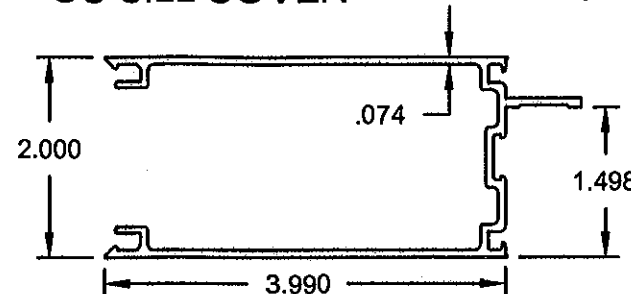
②① #8012 6063-T6 STILE
