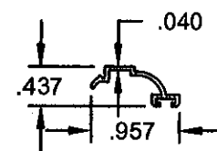
(108) #8024A 6063-T5 I.G. BEAD
