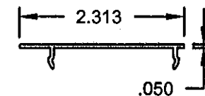
(62) #8029 6063-T5 SL JAMB TRIM
