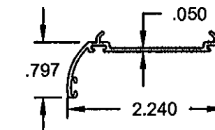
②④ #8016 6063-T5 BOTTOM SWEEP
