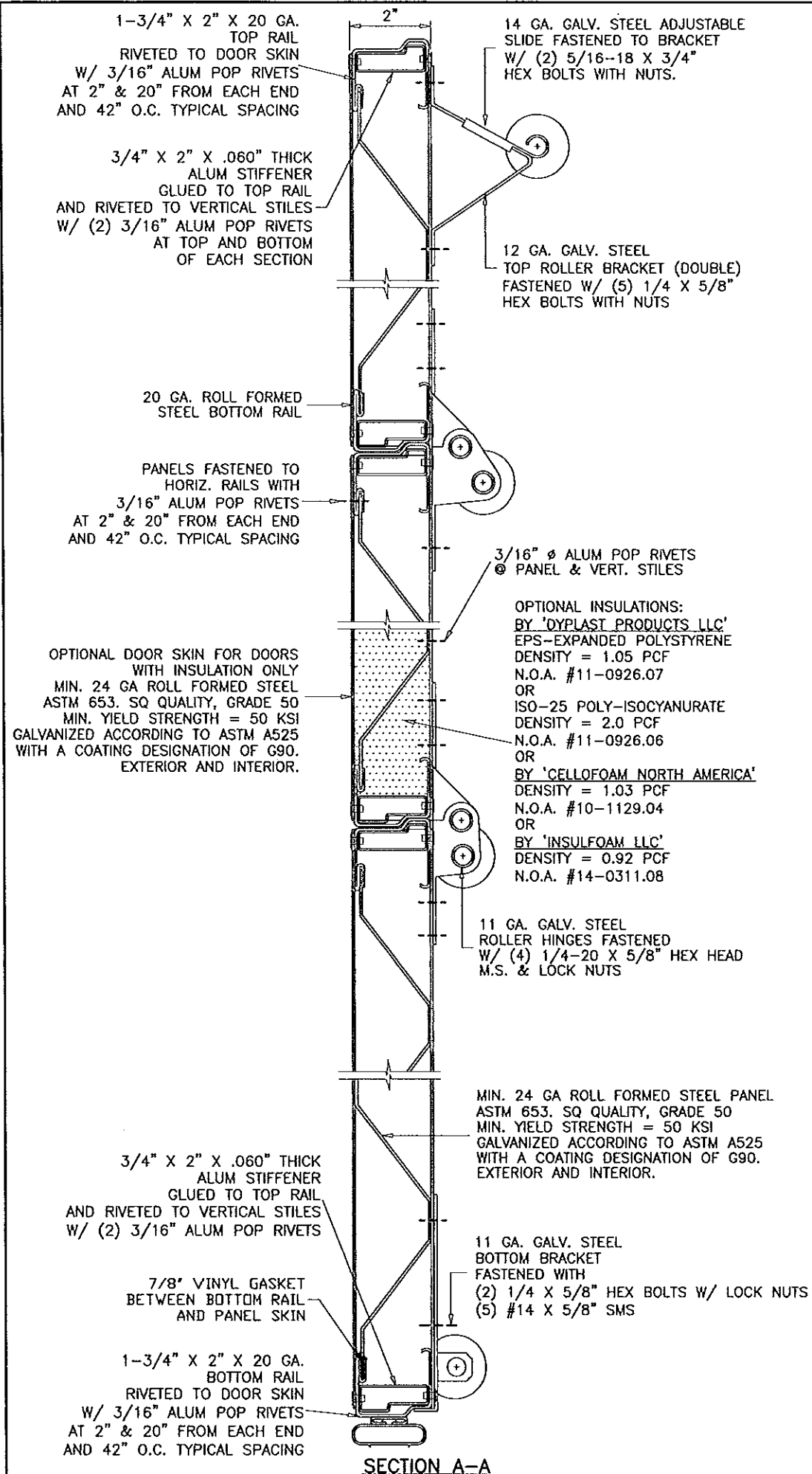
SECTION A-A
