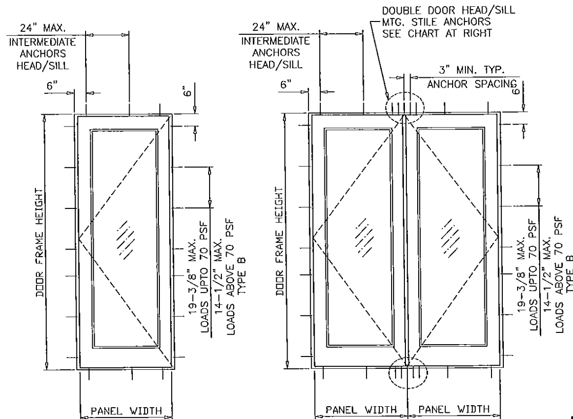
SINGLE DOOR OR SIDELITE
