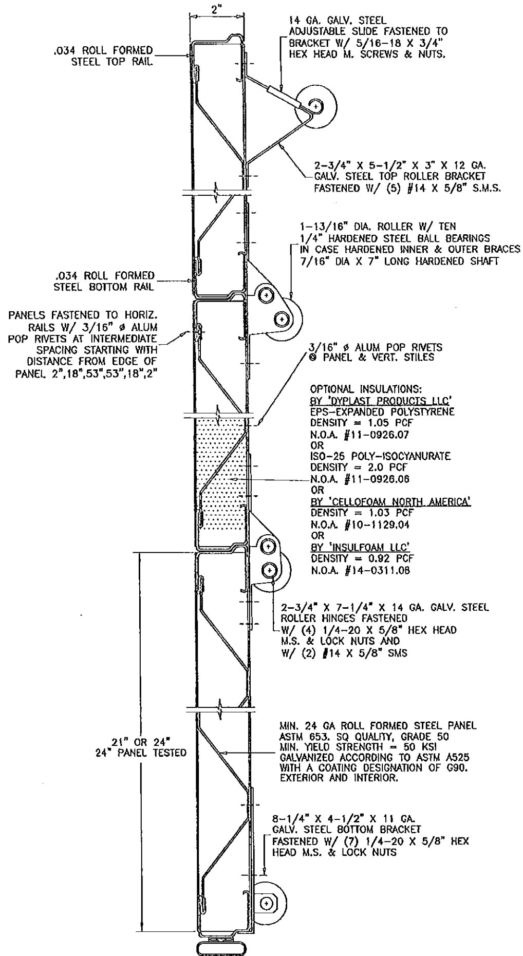
SECTION A-A
