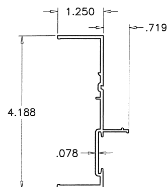
⑥ SIDELITE SLIP ON JAMB
