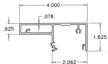
① DOOR FRAME HEAD/SILL
