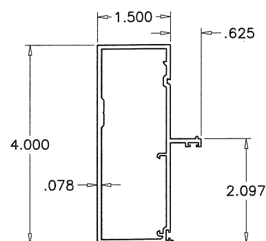
③ DOOR FRAME JAMB
