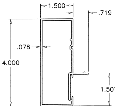
⑤ SIDELITE FRAME JAMB
