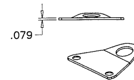
DOOR TOP LATCH OPPOSITE PART (KP-01-0149) (GALV. STEEL) (2 REQD.)
