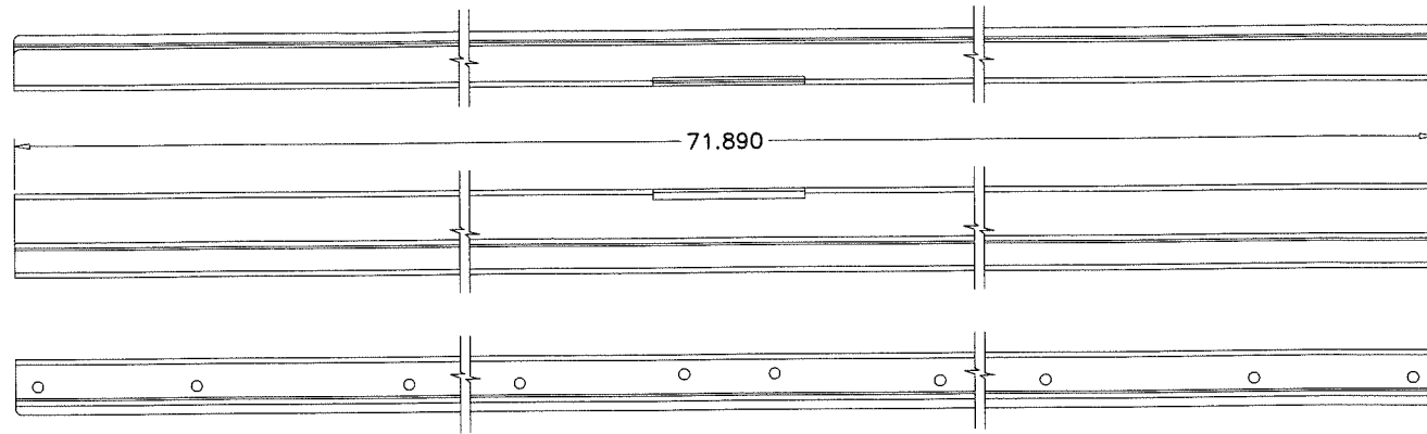
RIGHT DOOR STIFFENER (KP-01-0115) (GALV. STEEL) (1 REQD.)
