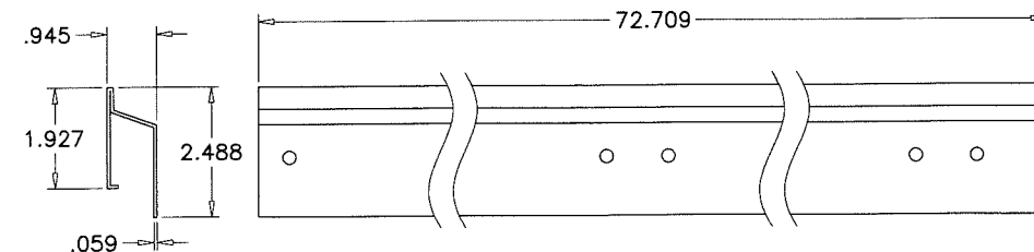
DOOR LATCH (-) (4 REQD.)
