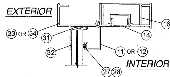
OPTIONAL HEAD FRAME
