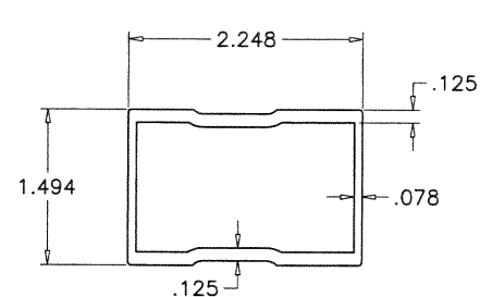
⑰ INTERLOCK STIFFENER
