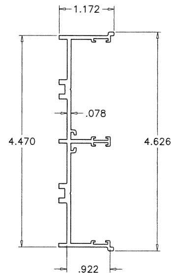
③ FRAME JAMB
