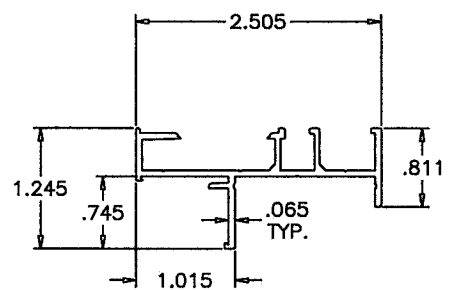
E1 FLUSH FRAME HEAD
