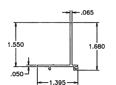
E11 NAIL FIN ADAPTER
