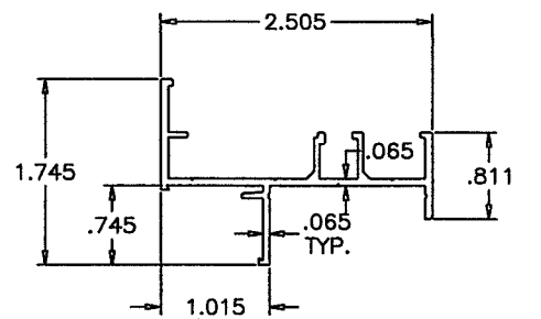
E12 FLANGE FRAME HEAD
