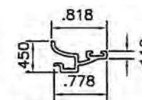
609-Glzg. Bead 6063-T5
