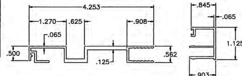
ALUMINUM BUCK 6063-T6
