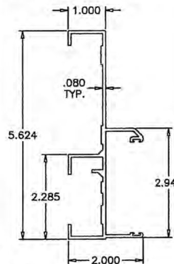
③ FRAME JAMB
