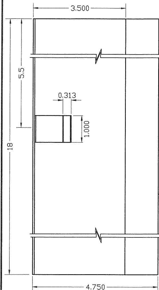
ELEVATION
