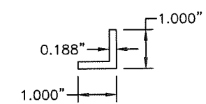
100 ANGLE N.T.S. 6063-T6
