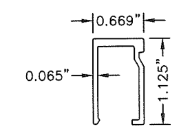
19 GLASS STOP N.T.S. 6063-T6
