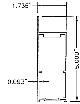
7 TOP RAIL, SO N.T.S. 3000 6063-T6
