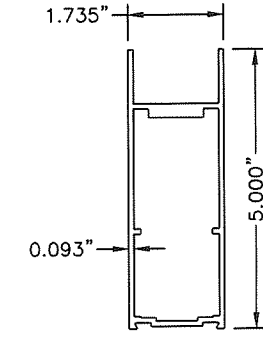
8 TOP RAIL, O N.T.S. 2000 6063-T6
