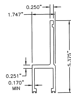
26 HANGER N.T.S. 6063-T6
