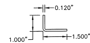
48 BRACKET N.T.S. 6063-T6
