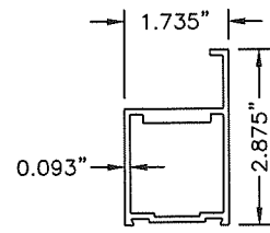
10 TOP RAIL, SX N.T.S. 2000 6063-T6
