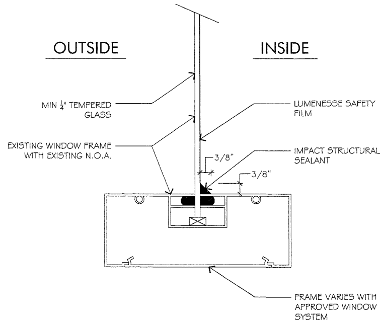
1 GLAZING DETAIL 1 SCALE: 1" = 1'-0"
