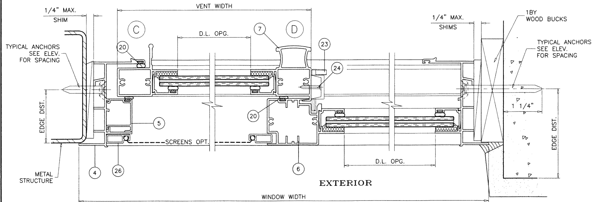
XO LAYOUT
