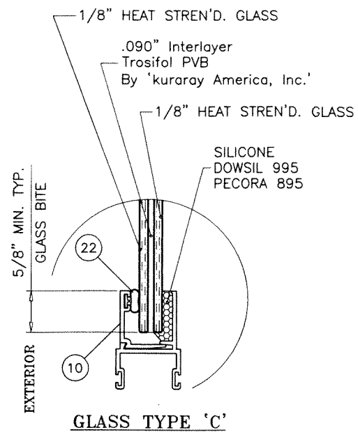
GLAZING OPTIONS
