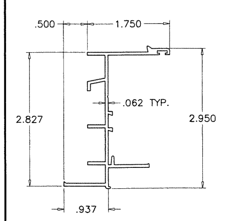
4 FRAME JAMB
