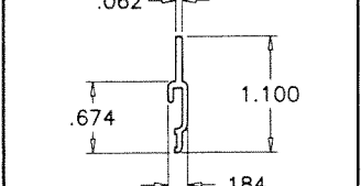
13 SILL RISER
