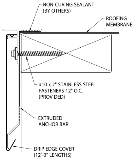
VERSiTRIM 2000 DRIP EDGE
