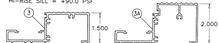
STD. SILL
