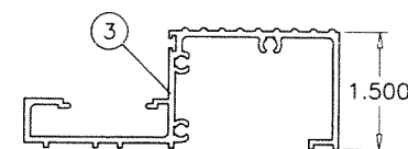
STD. SILL
