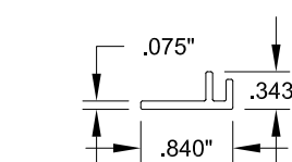
17 ADD-ON FIN/FLANGE #20008, Rigid PVC
