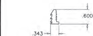
6 WEDGE GASKET
