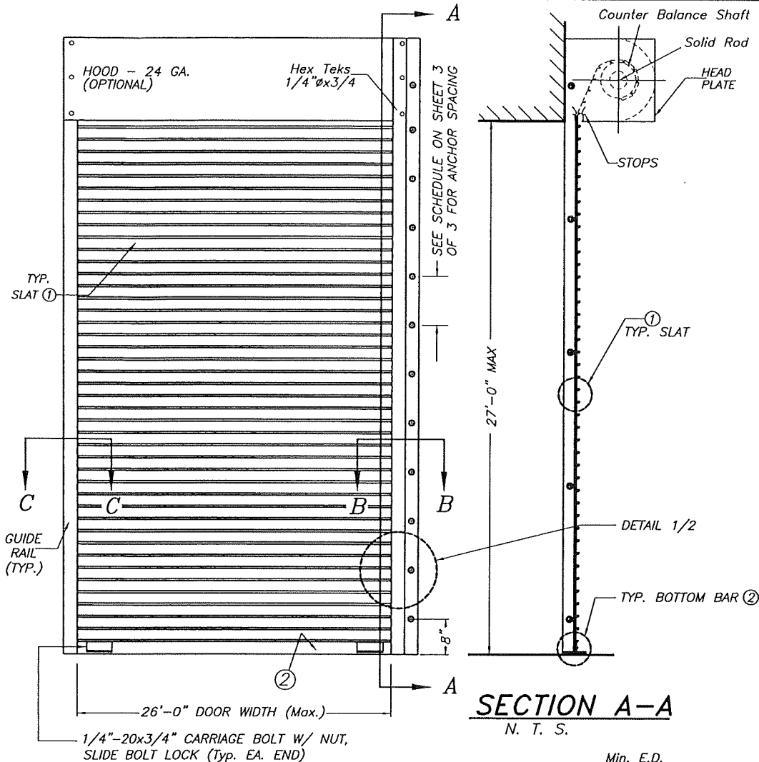
TYPICAL DOOR ELEVATION N. T. S.
