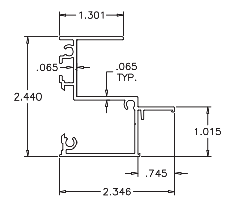
E3 FLUSH FRAME JAMB
