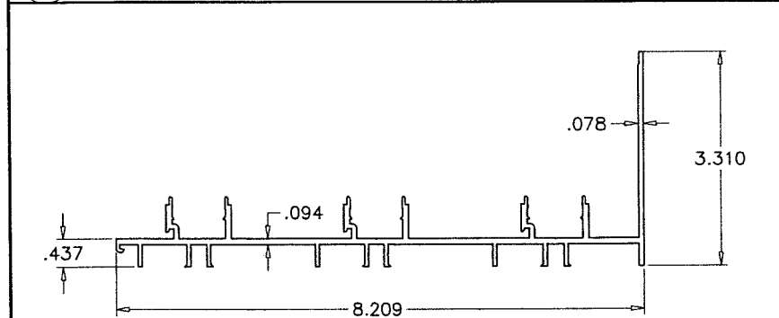
E15 FRAME SILL
