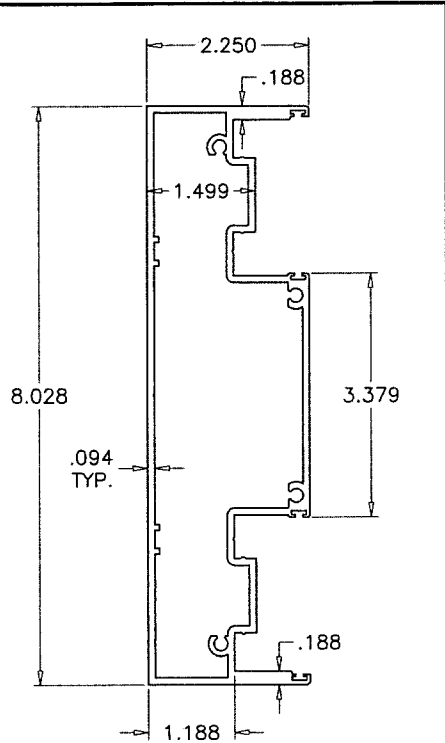
E16 STD. FRAME JAMB
