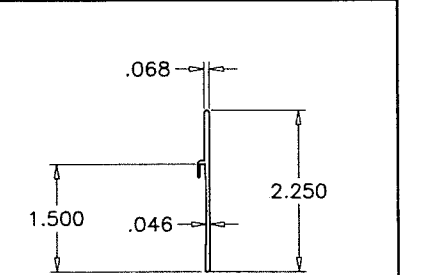
E20 SILL RISER
