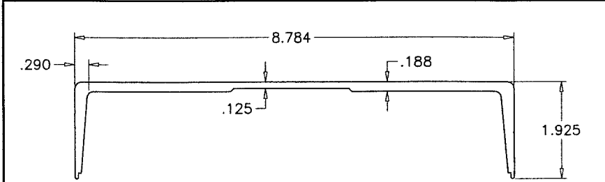
E18 RECEPTOR STIFFENER
