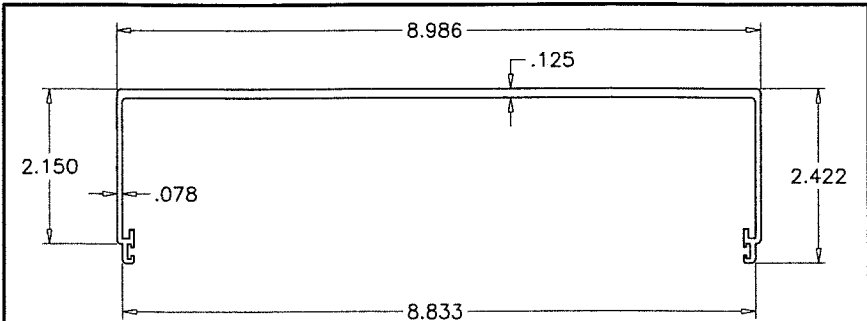
E17 HEAD RECEPTOR
