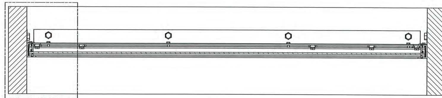
SECTION BH-BH N.T.S.
