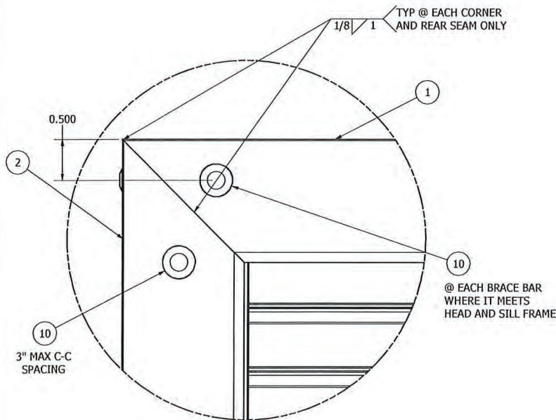
4 2 CORNER CONNCTION DETAIL N.T.S.
