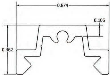
ITEM 3 BRACE BAR N.T.S. RUSKIN PART #RSM314
