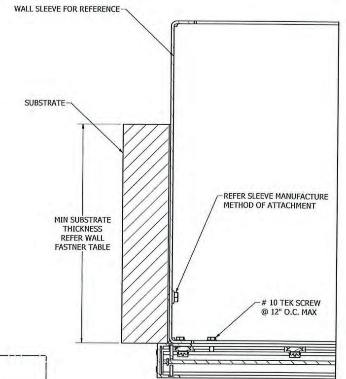
DETAIL CV N.T.S.
