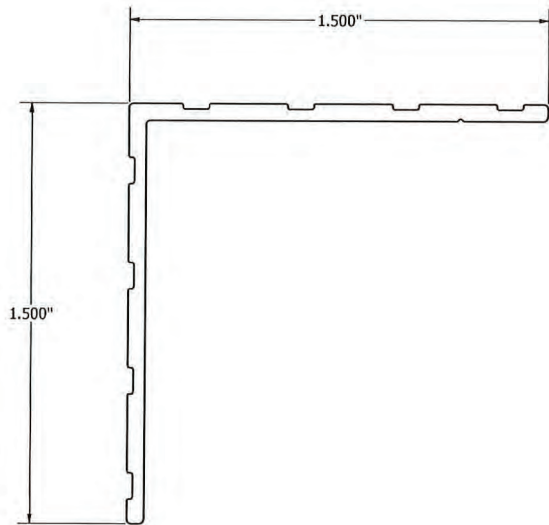
ITEM 5 CORNER LUG N.T.S. RUSKIN PART # 285
