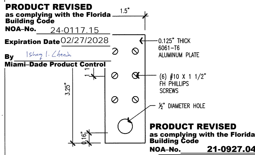
K WINDOW MULLION SCALE: 6"=1'-0"
