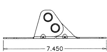
#4 HINGE (11 GA. STEEL)
