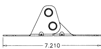
#5 HINGE (11 GA. STEEL)
