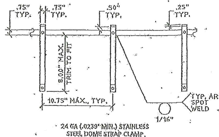
6 DOME CLAMP STRAP SCALE: 1-1/2" = 1'-0"
