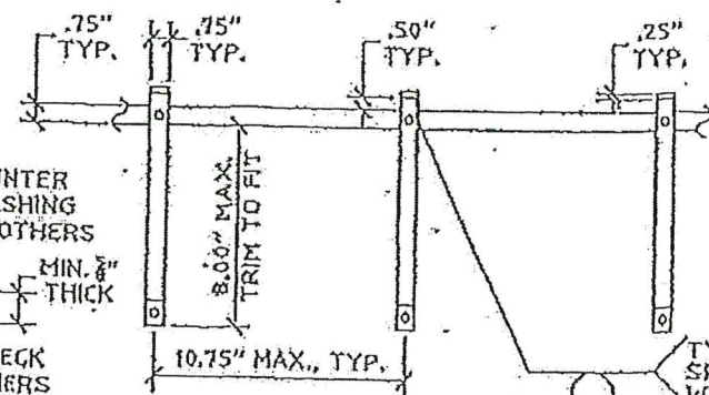
⑤ DOME CLAMP STRAP SCALE: 1-1/2" = 1' - 0"
