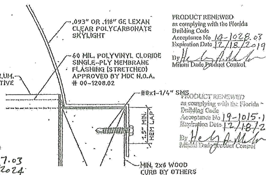
6 60 MIL. MEMBRANE FLASHING DETAIL SCALE: HALF SIZE
