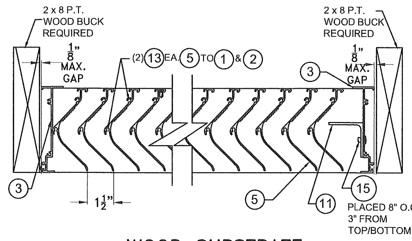
WOOD SUBSTRATE N.T.S.
