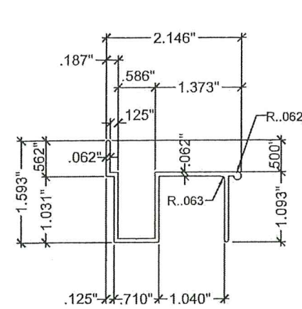
(D) FLOOR SILL SPA007
