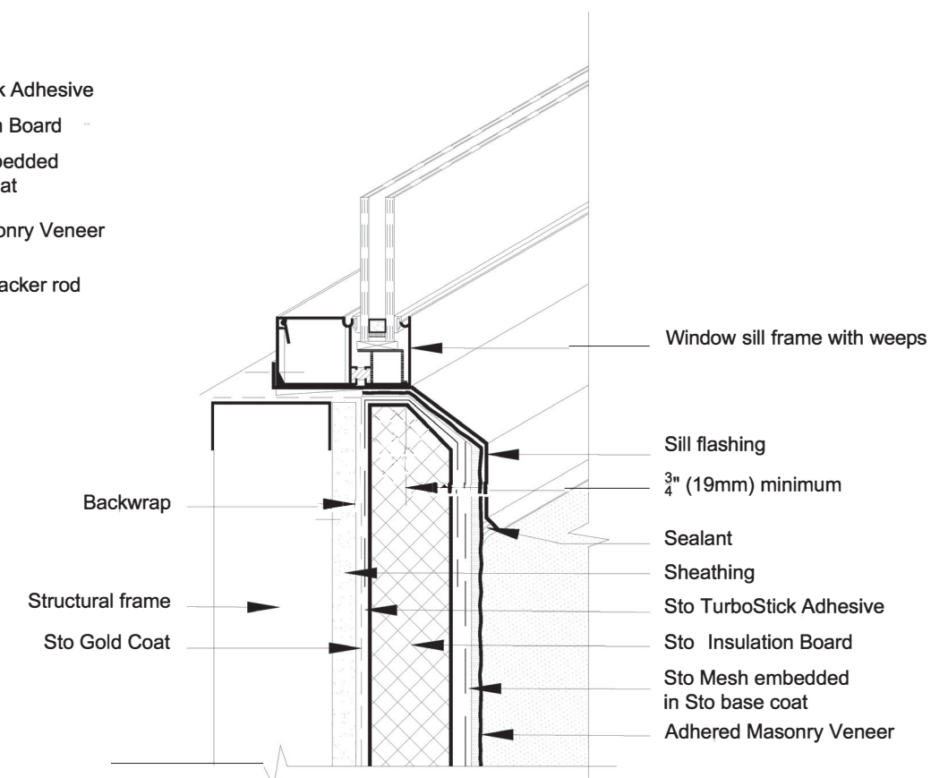
WINDOW SILL N.T.S.
