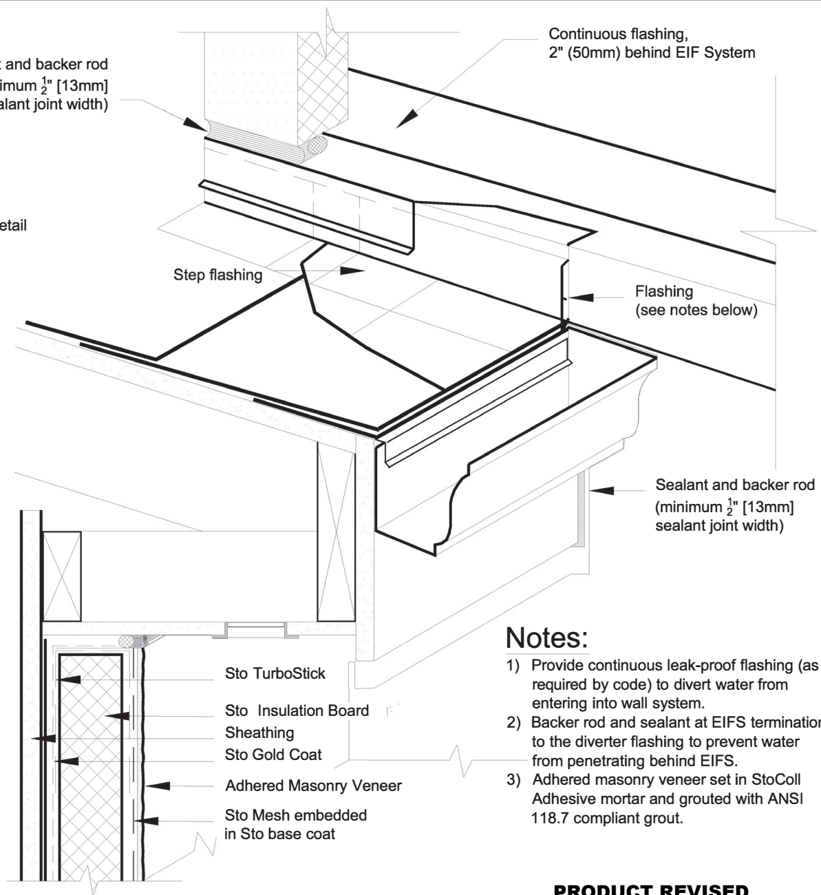
OVERHANG N.T.S.
