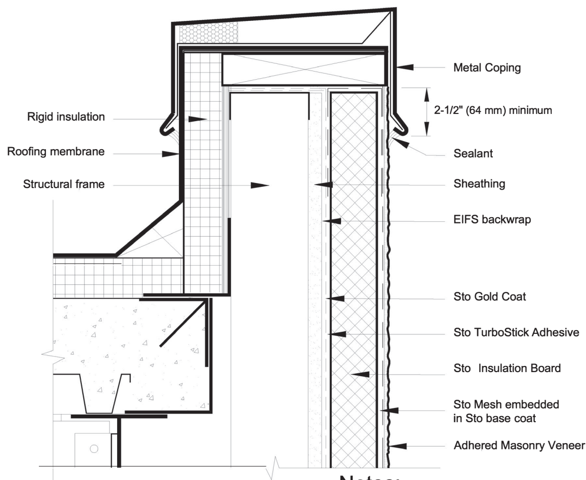
PARAPET N.T.S.
