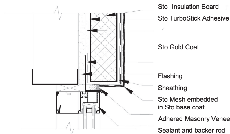
WINDOW HEAD N.T.S.
