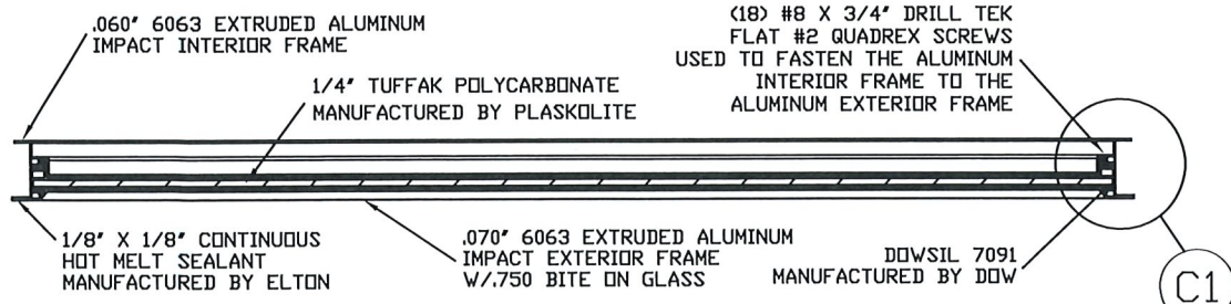
SECTION C-C IMPACT WINDOW DETAIL N.T.S.
