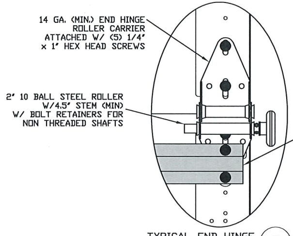
TYPICAL END HINGE N.T.S.
