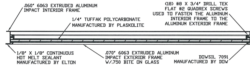
SECTION C-C IMPACT WINDOW DETAIL N.T.S.
