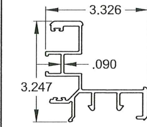
㊶ 90° CORNER ASTRAGAL
