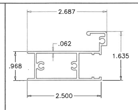
(E5) JAMB STILE
