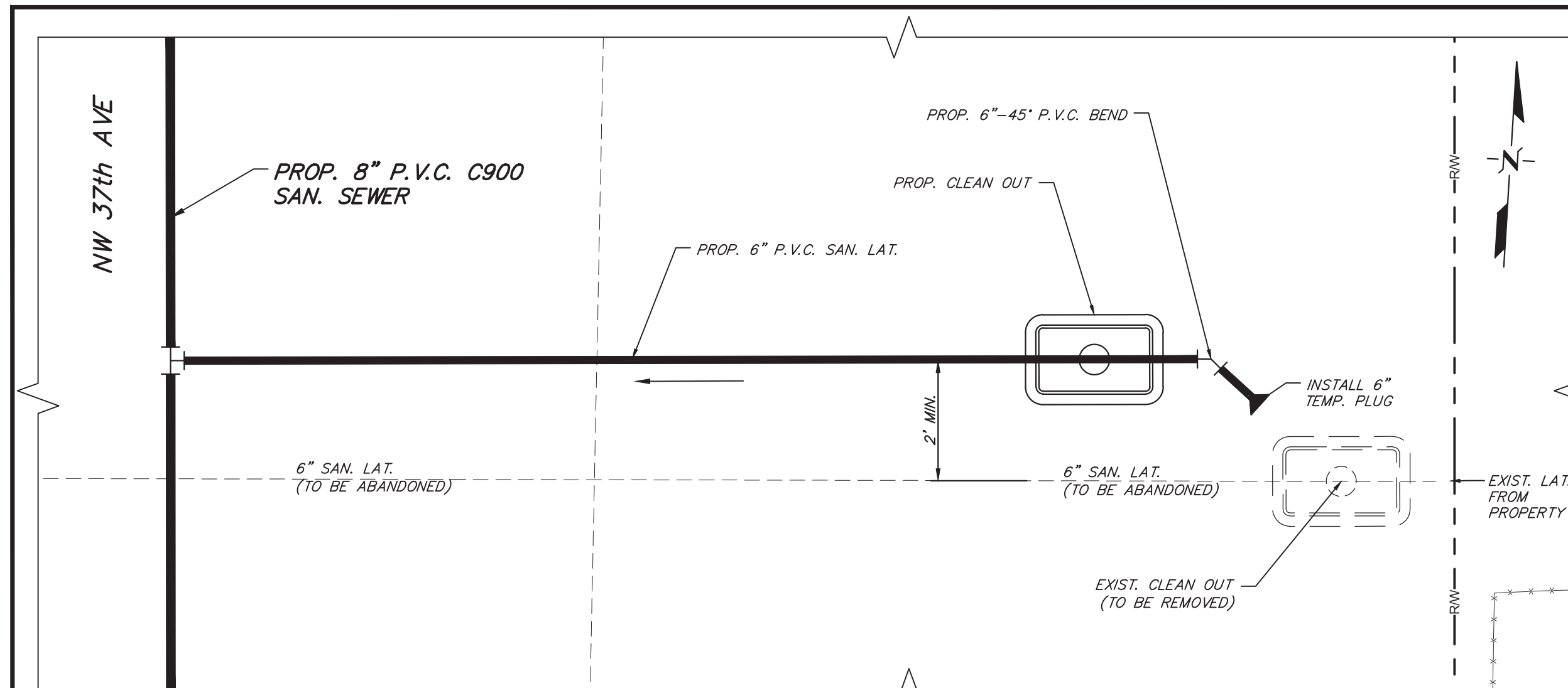
PHASE A SCALE: 1"=2'
