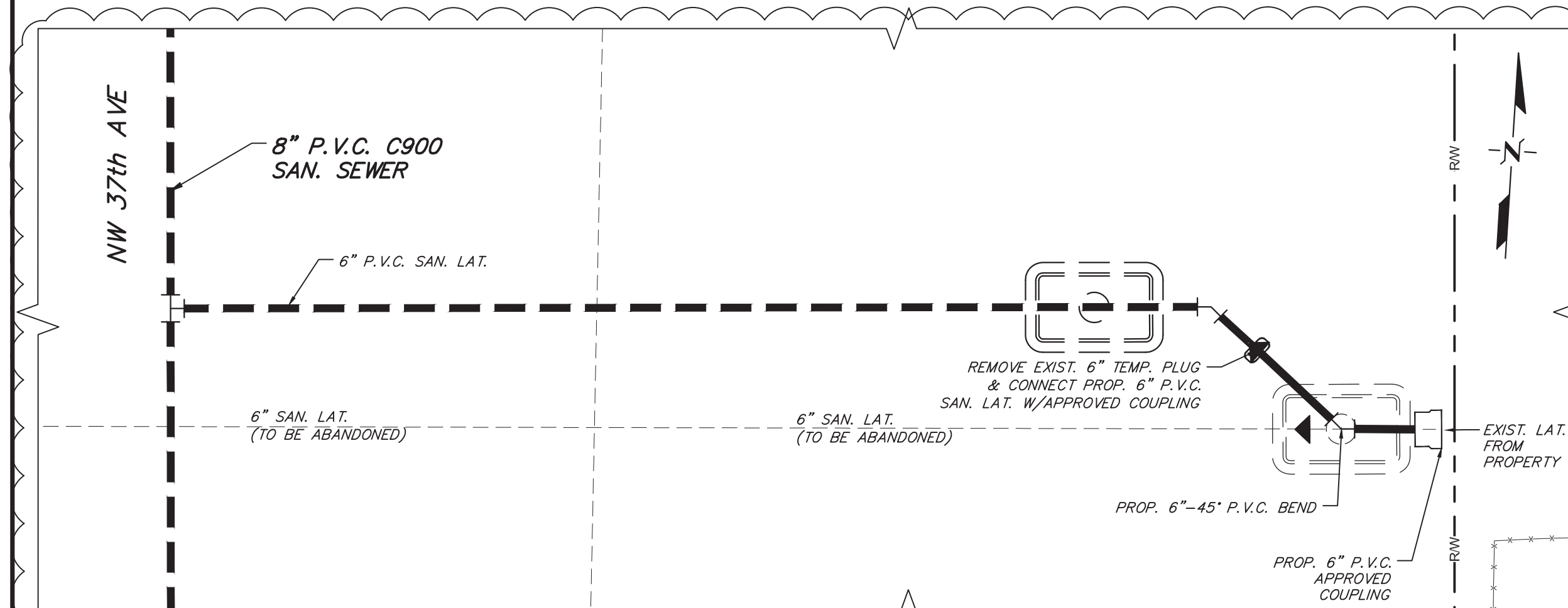
PHASE A SCALE: 1"=2'
