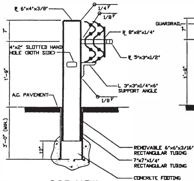
SIDE VIEW N.T.S.
