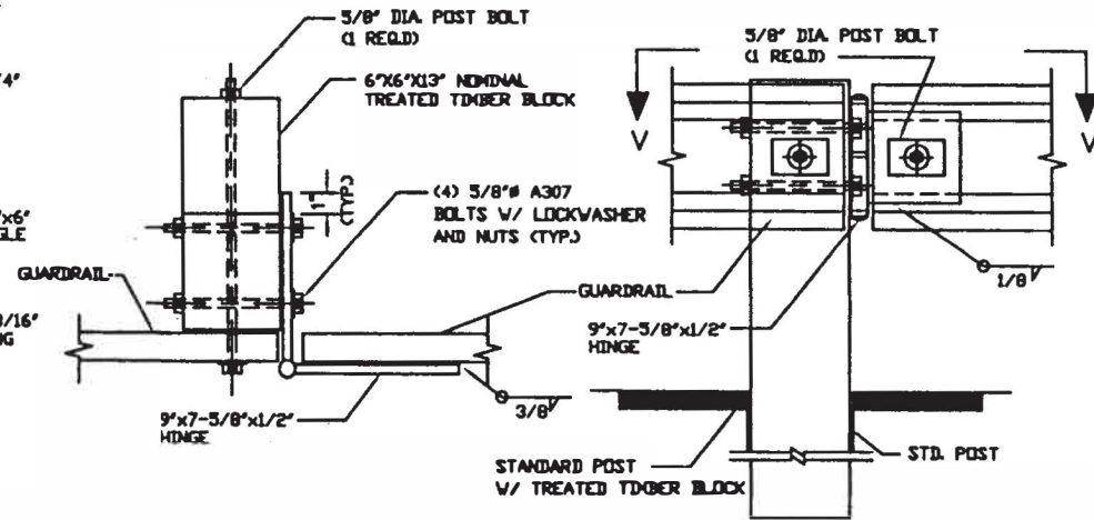
SECTION "V - V" N.T.S.
