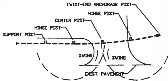
ACCESS GATE PLAN N.T.S.
