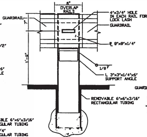
FRONT VIEW N.T.S.
