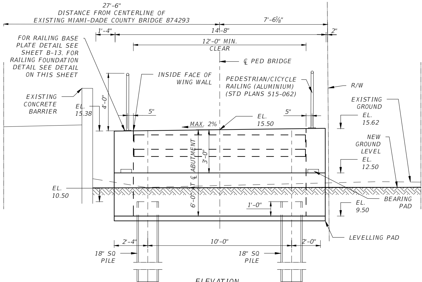
ELEVATION
