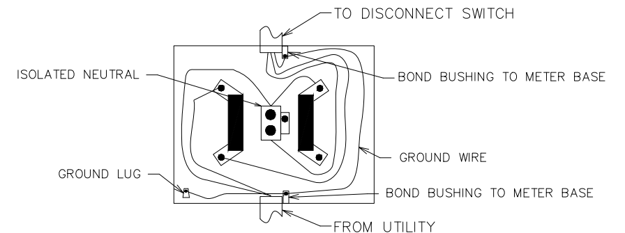
METER SOCKET DETAIL
