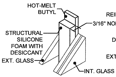
㉖ SUPER SPACER ® NXT ™
