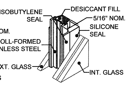
㉘ XL EDGE ™ SPACER
