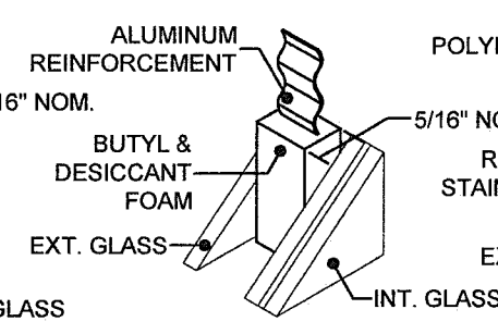
㉗ DURASEAL ® SPACER
