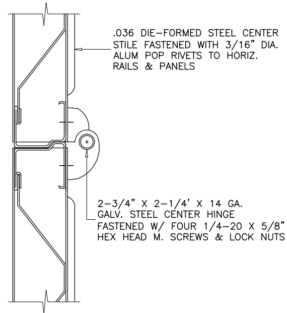
SECTION D-D
