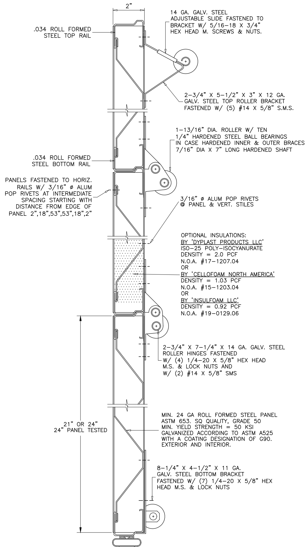
SECTION A-A
