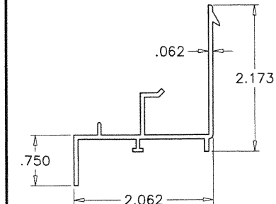
SILL C-3002 6063-T6
