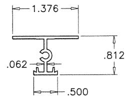
HORIZ. MUNTIN C-3010 6063-T6
