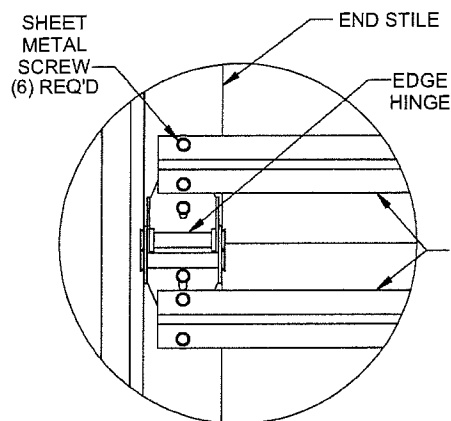
EDGE HINGE / U-BAR DETAIL
