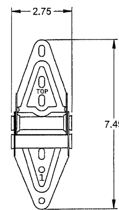
EDGE HINGE .086 GALV. STEEL
