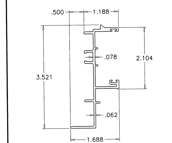
④ MOV. FRAME JAMB
