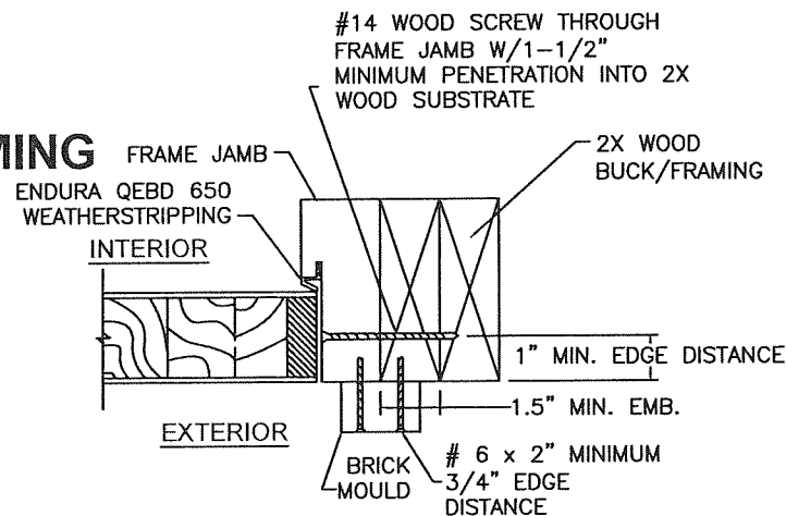
7 JAMB ANCHORAGE
