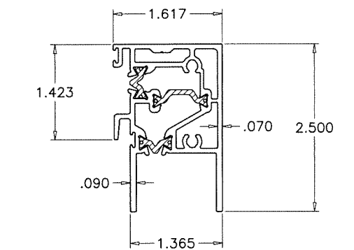
E10 VENT TOP RAIL
