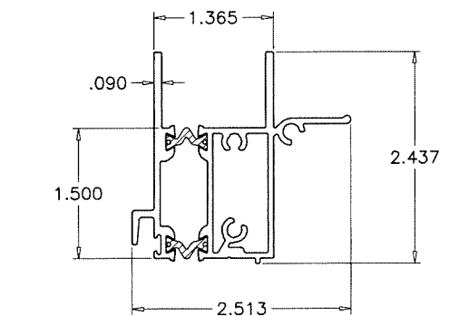
E11 VENT BOTTOM RAIL
