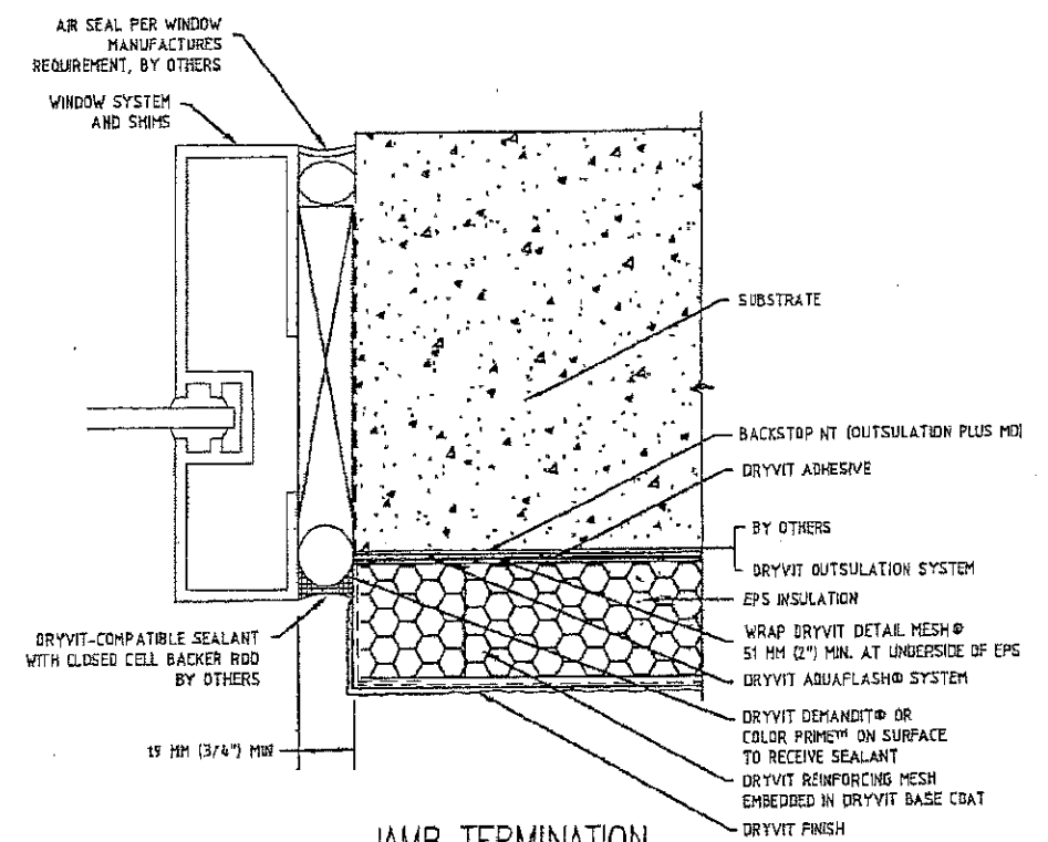
JAMB TERMINATION
