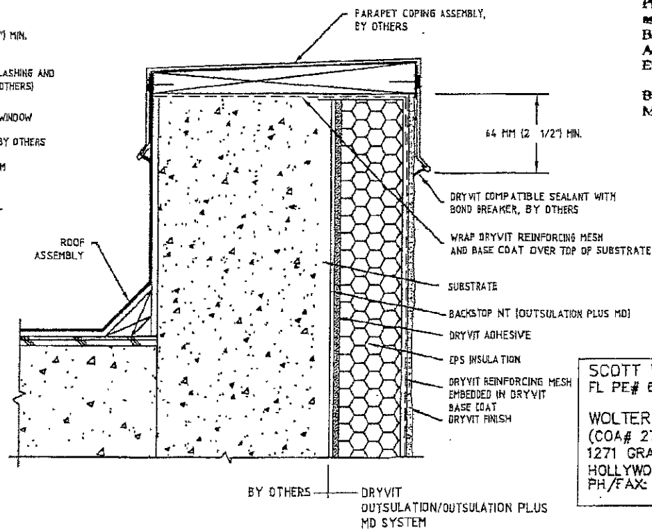
PARAPET
