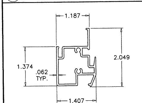
E8 FIX. MEETING RAIL
