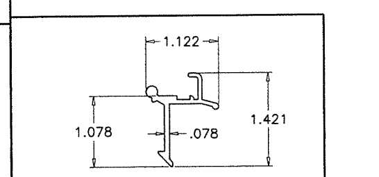
E10 GLAZING BEADS
