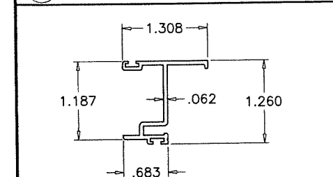
E7 VENT SIDE RAIL
