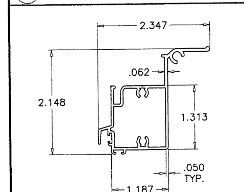
E6 VENT BOTTOM RAIL
