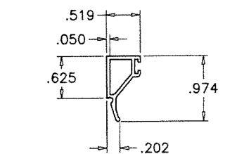
E10A GLAZING BEADS
