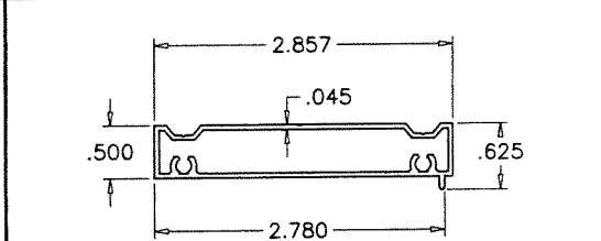
E12 FLUSH FRAME ADAPTER
