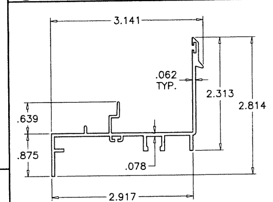
E2 FRAME SILL (STANDARD)
