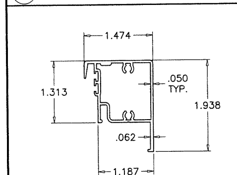
E5 VENT TOP RAIL
