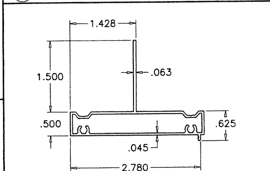
E15 FLUSH FRAME ADAPTER WITH FIN
