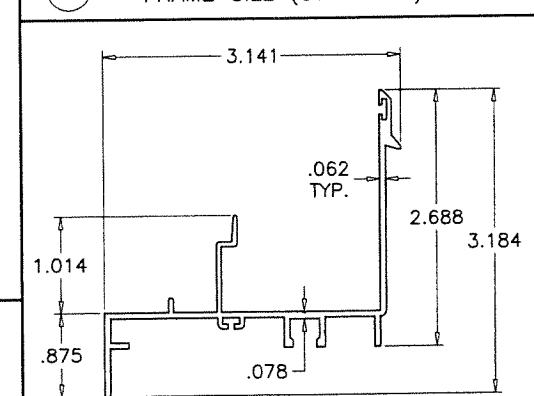
E3 FRAME SILL (HI-RISE)
