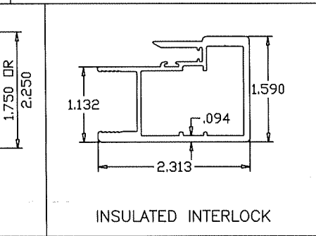
ASTRAGAL STILE
