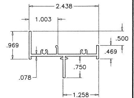
FRAME JAMB GOP-7
