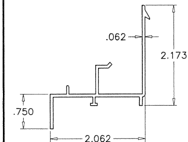
2 SILL 6063-T5
