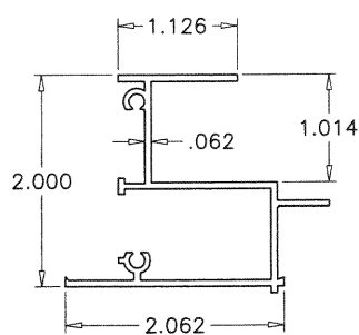
3 FRAME JAMB 6063-T6
