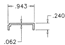
17 SHEAR CLIP 6063-T6
