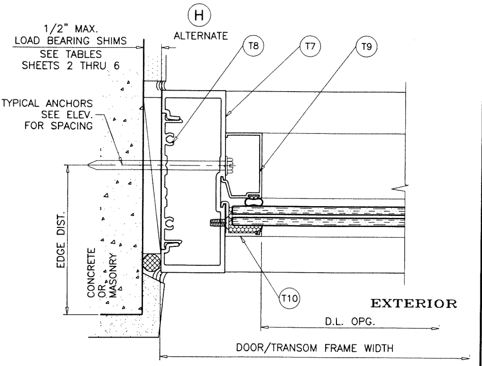
TRANSOM JAMB SERIES-8000 FRAMES OPTION
