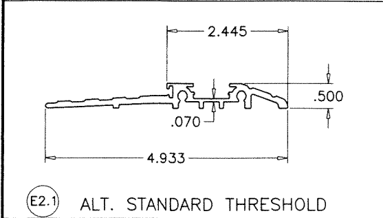
E2 STD. THRESHOLD ES9014
